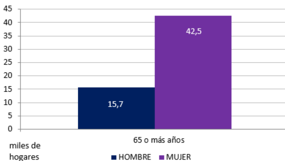
FIGURA 1: Personas de 65 y más años que viven solas en Asturias, por sexo. 2019
